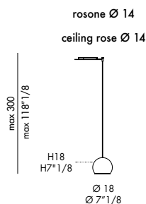
CHERRY_1 sospensione CHERRY_1 pendant
